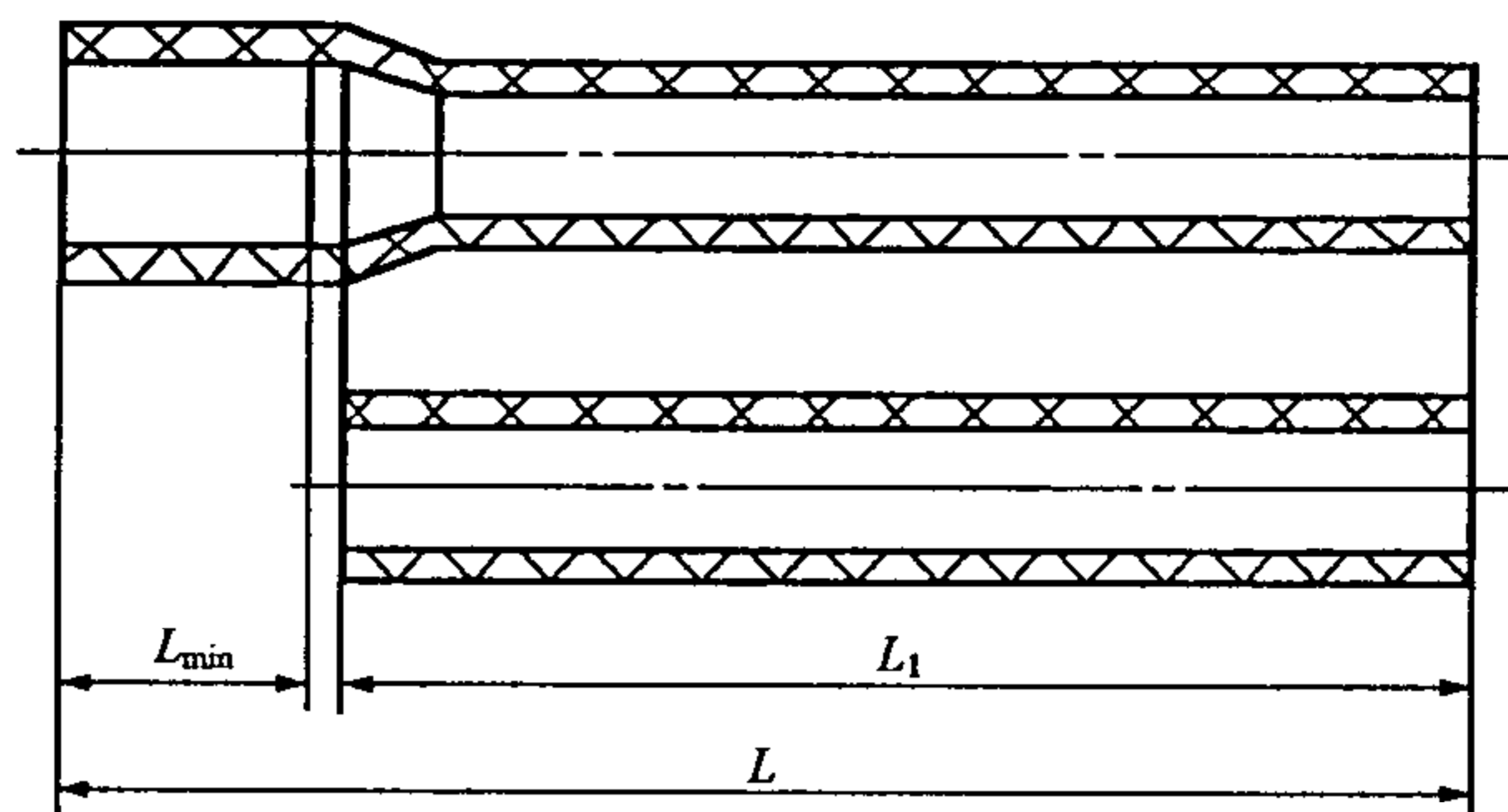
图 1 管材长度示意图
