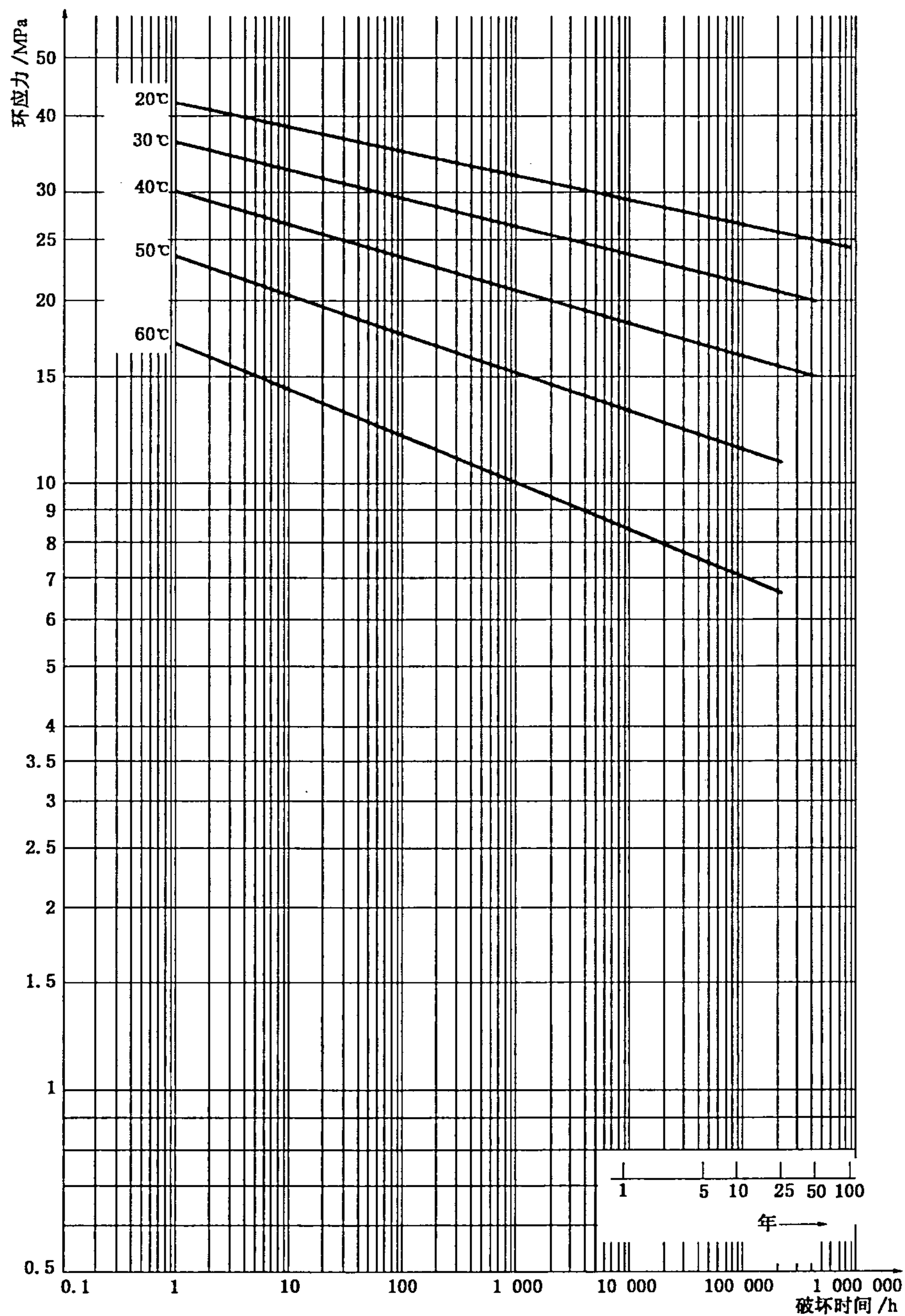
图 A.1 PVC-U 预测静液压强度参照曲线
